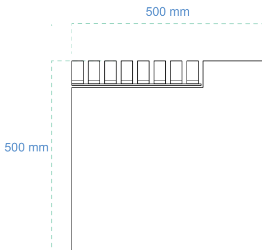
FRONT - Modul med betonkant
